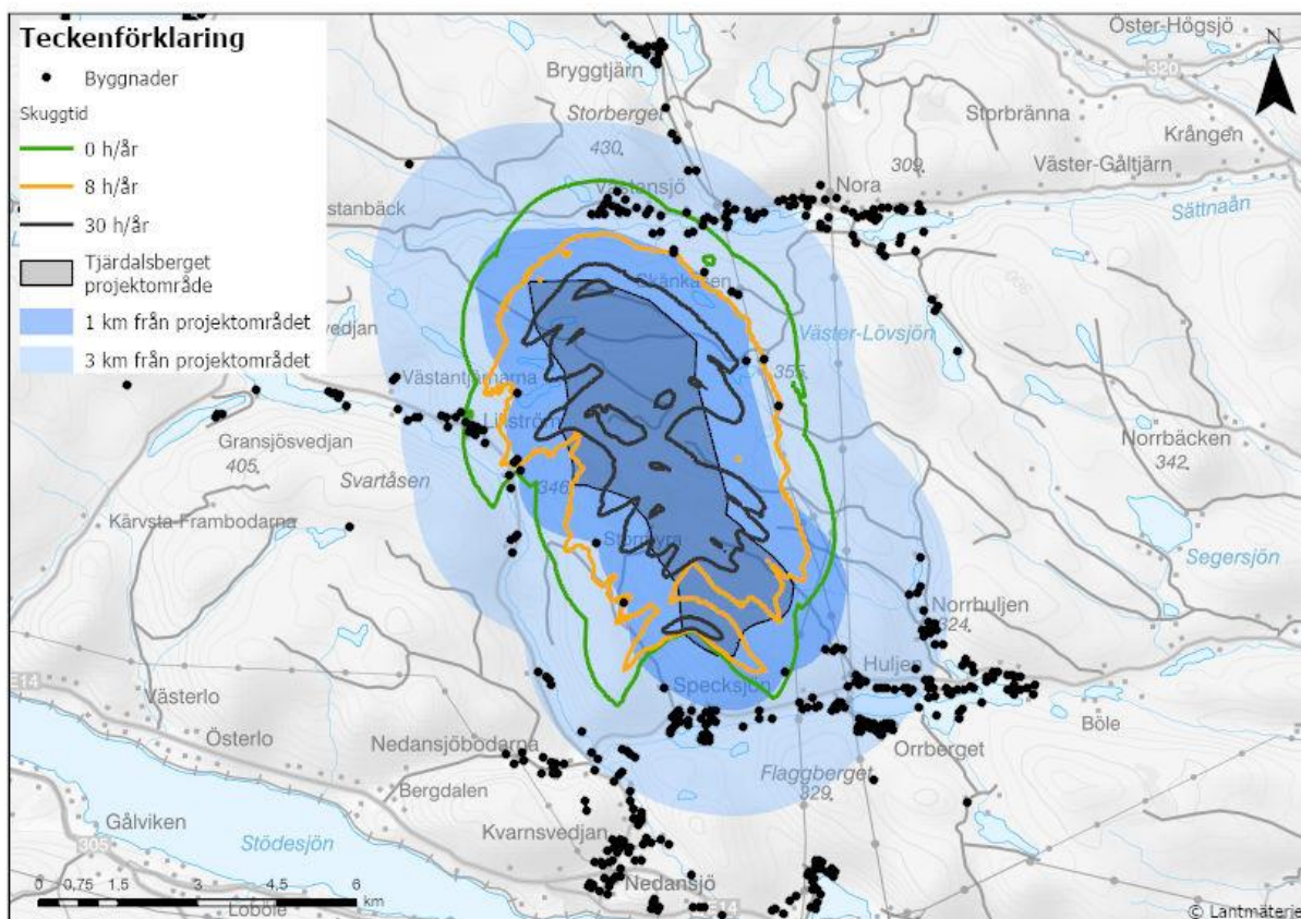
Figur 14. Skuggberäkning baserad på exempellayouten för Tjärdalsberget.
