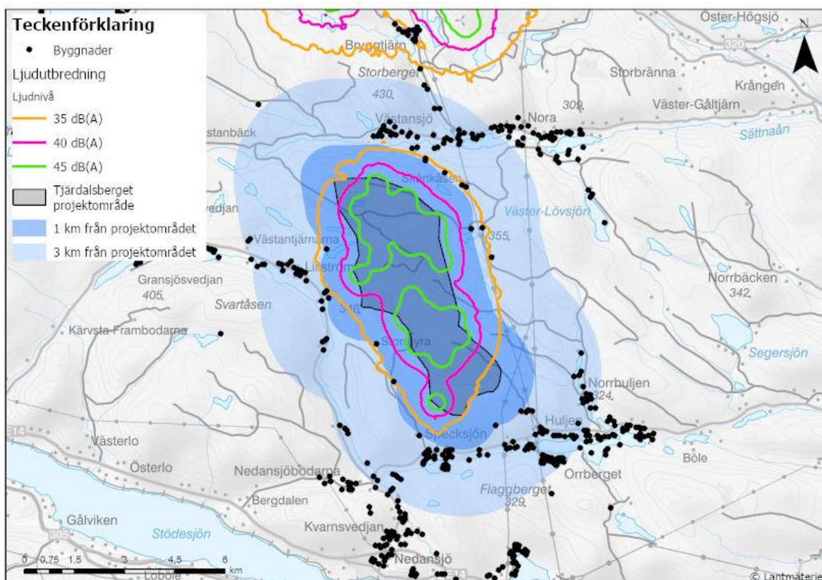
Figur 13. Ljudutbredning baserad på exempellayouten för Tjärdalsberget. Norr om Tjärdalsberget syns ljudutbredningen från Nylandsbergens vindkraftsanläggning som är uppförd sedan tidigare.
