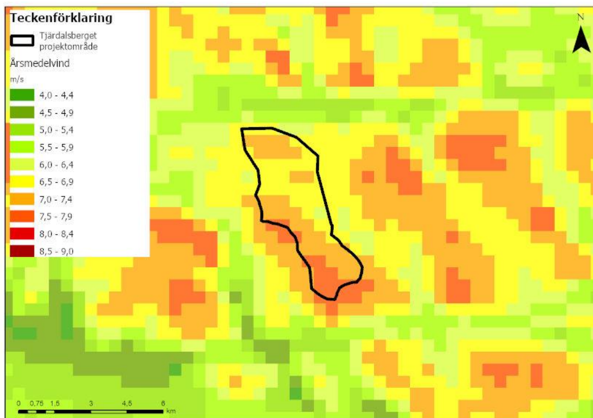
Figur 9. Vindanalysmodellering som visar att årsmedelvinden inom projektområdet för Tjärdalsberget på 140 meters höjd är 6,4 - 7,9 meter per sekund.
